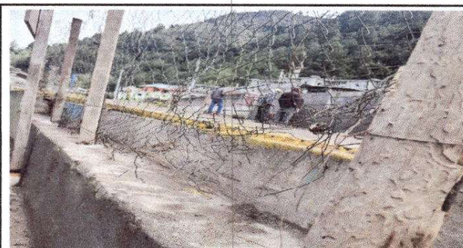
Foto 6: Reparación de muro perimetral de block con tubo hg y malla galvanizada, soleras intermedias y columnas
